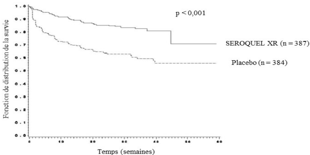
Figure 2 : Délai écoulé jusqu'à la survenue d'un épisode dépressif; essai à répartition aléatoire à plus long terme portant sur le sevrage; courbes de Kaplan-Meier (population en intention de traiter [ITT])
